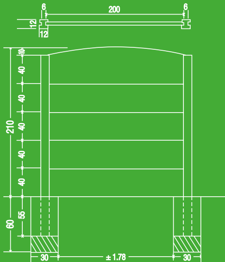
Afmetingen voor een hout- of steenmotiefplaat
